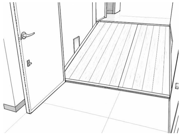
④から⑤への動線上の仮設スロープ
